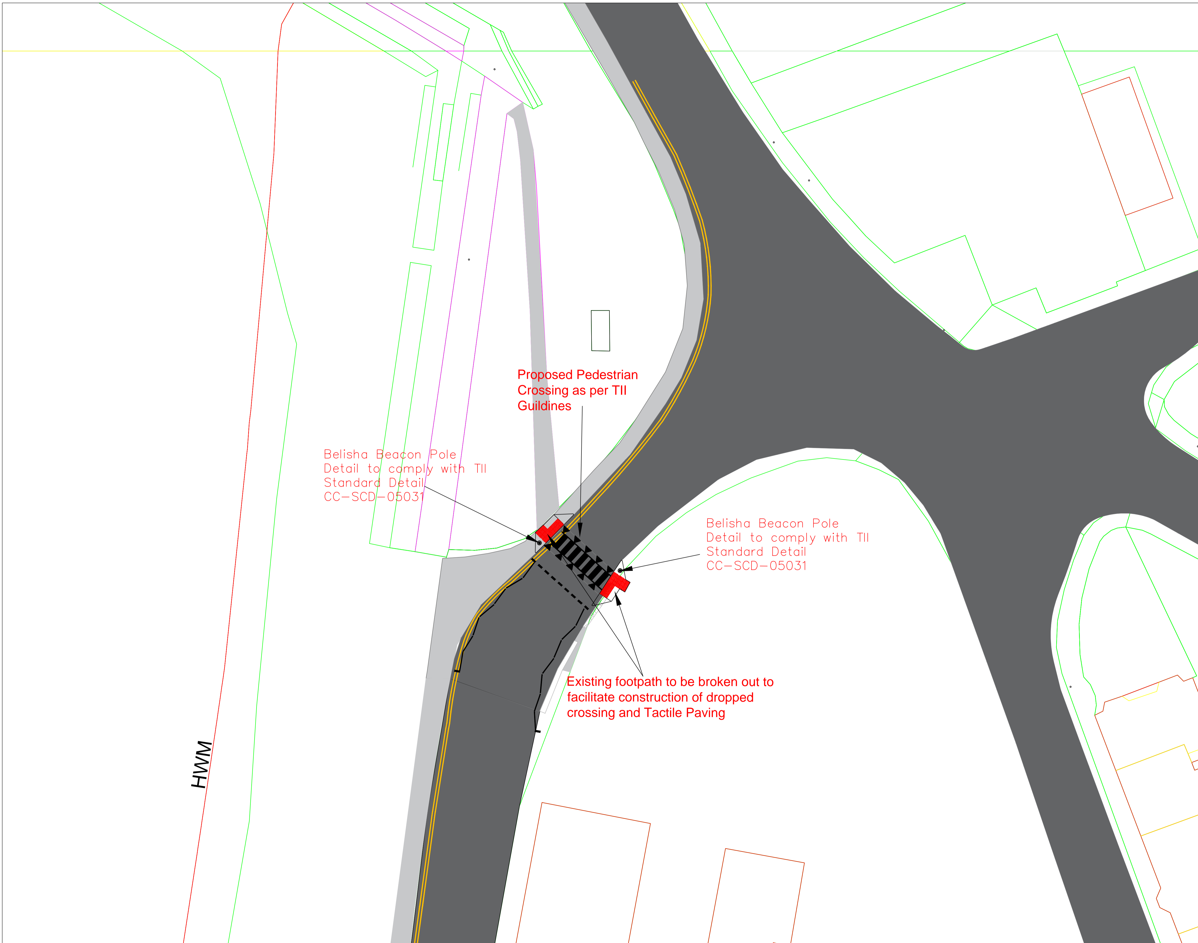
SITE LOCATION MAP SCALE: 1/200 @ A1
